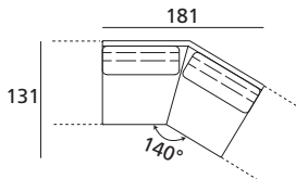
Angolo sagomato da 181x131 Shaped corner 181x131
